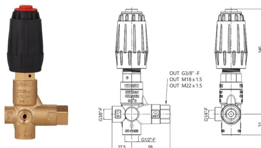
型 号 流 量 最大压力 额定温度 进水口 出水口 回水口 重量 Model Flow Pressure Temperature inlet Outlet Backwater Weight L/min gpm bar psi ℃ thread thread By-pass KG VB350 40.0 10.5 350 5075 90 G3/8" G3/8" G1/2" 0.9 VG350 40.0 10.5 350 5075 90 G3/8" G3/8" G1/2" 1.1
