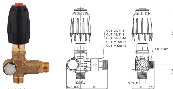
型 号 流 量 最 大 压 力 额定温度 进水口 出水口 回水口 重量 Model Flow Pressure Temperature inlet Outlet Backwater Weight L/min gpm bar psi ℃ thread thread By-pass KG VW30 A 40.0 10.6 300 4350 90 G3/8" G1/2" G1/2" 0.55 VW30 B-D 50.0 13.2 300 4350 90 G1/2" G3/8" G1/2" 0.65
